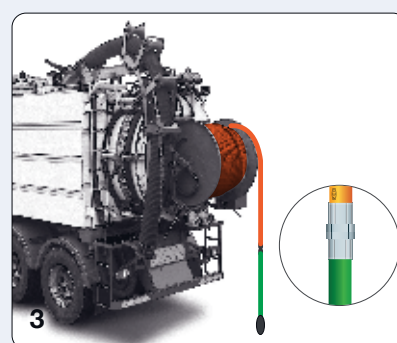
Rubber or thermoplastic "Leader Hose"; to facilitate the operation and to signal the nozzle return. Tubo Leader di gomma o termoplastico che faciliti l'operazione di inserimento e segnali l'uscita dell'ugello durante il recupero del tubo.
