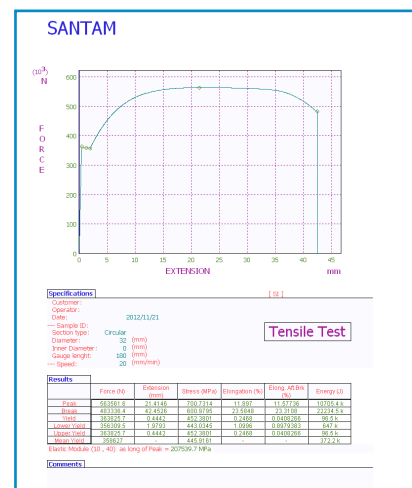
گزارش تست کشش آرماتور با اکستنسومتر
