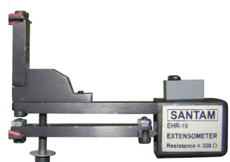
اکستنسومتر کورس کوتاه EHR10
