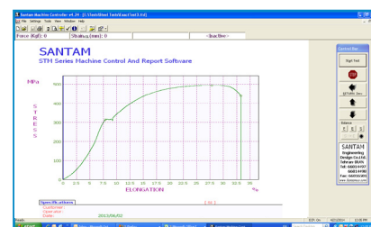
تست کشش بدون اکستنسومتر
